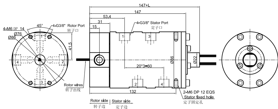
MK43S-S12(S18,S24,S36) 尺寸图 4进4出G3/8"牙+12~36路信号(2A)
