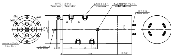
MAPH400-03 尺寸图
